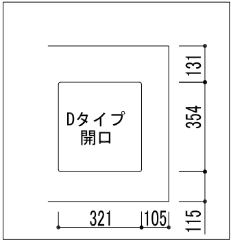
天板開口 Dタイプの場合
