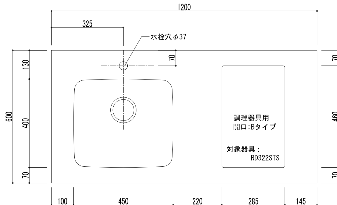
平面図
