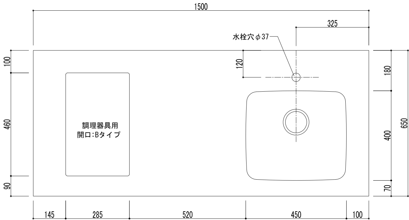
平面図
