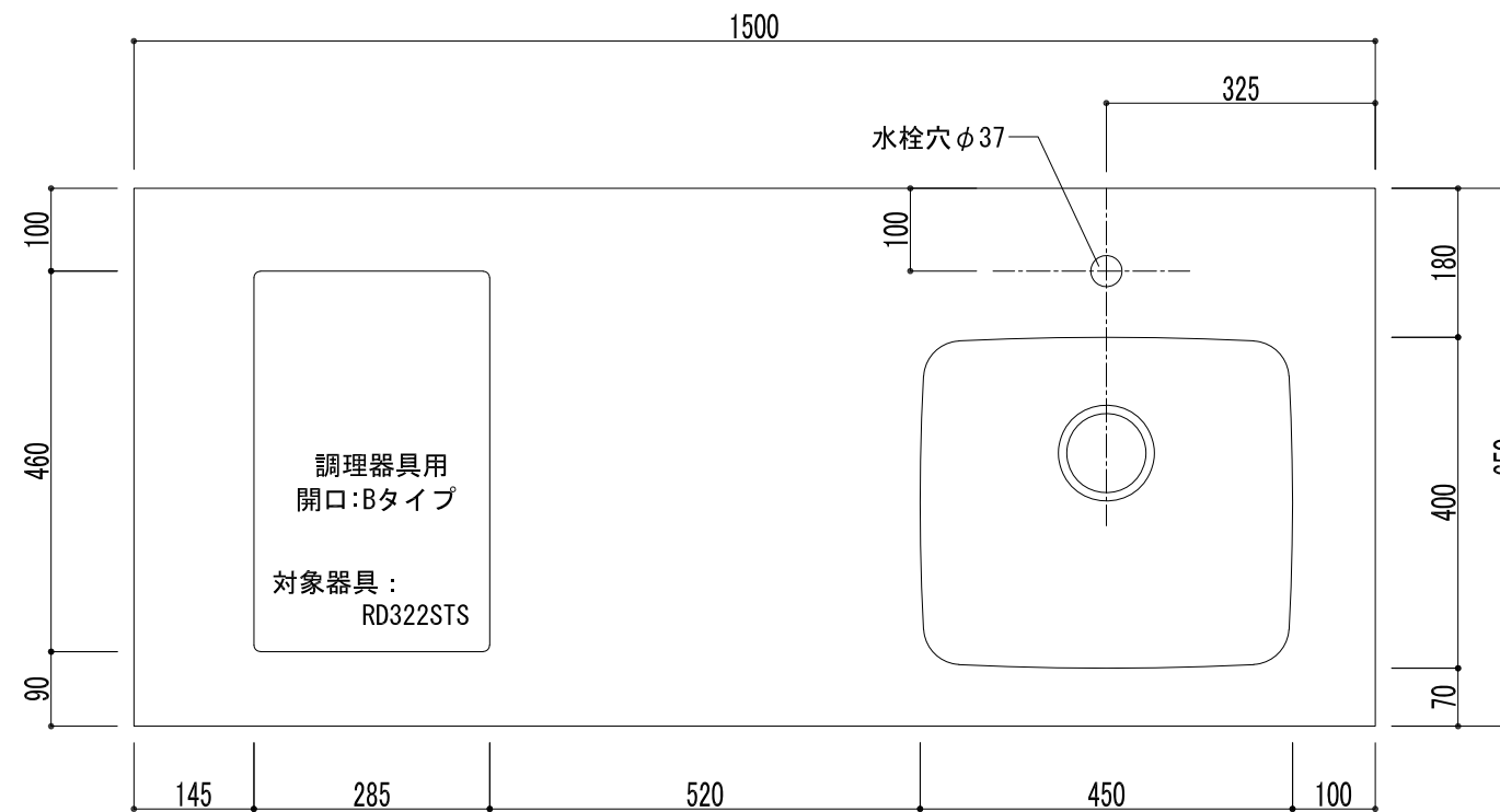
平面図
