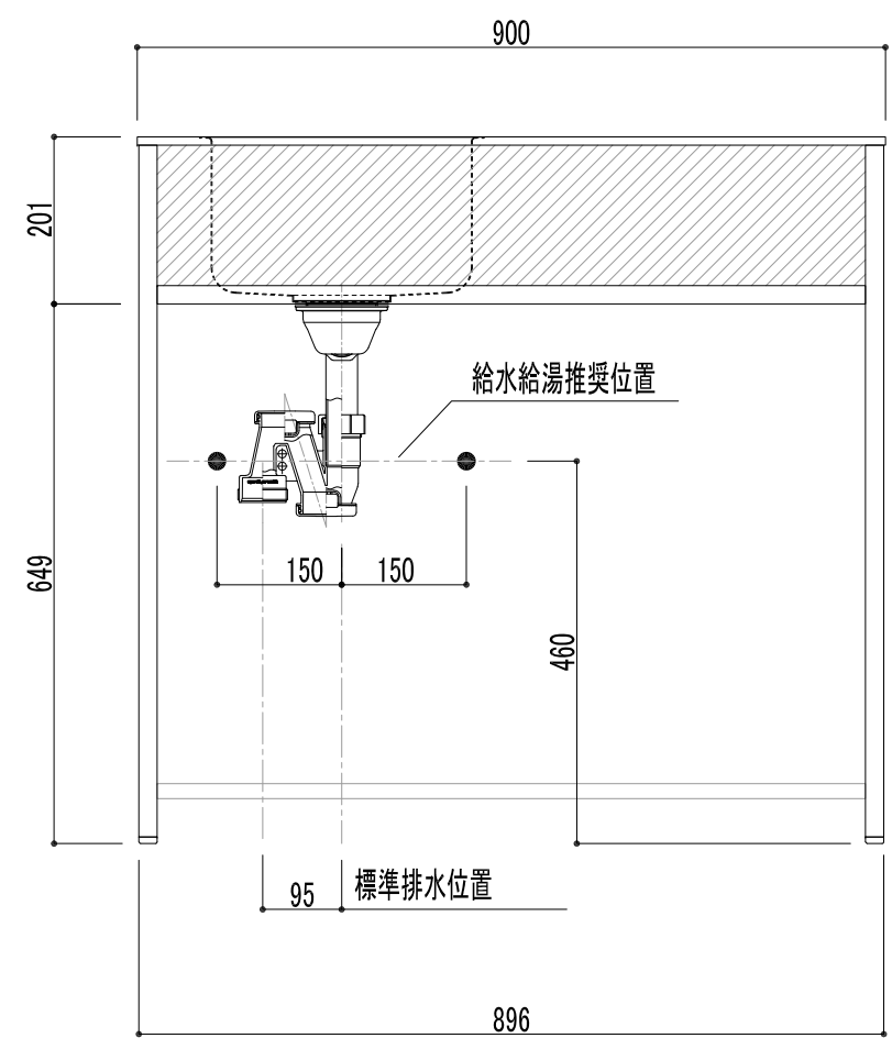
正面図
