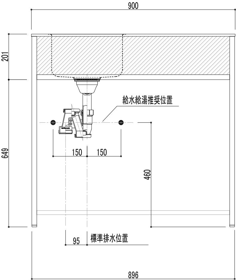
正面図
