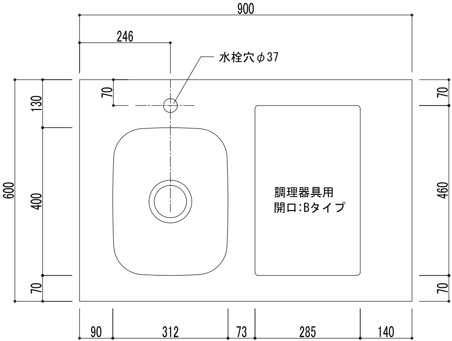
平面図
