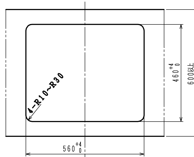
ワークトップ穴開け寸法
