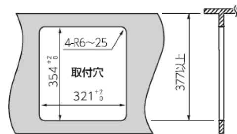
取付開口寸法
