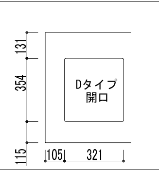
天板開口 Dタイプの場合
